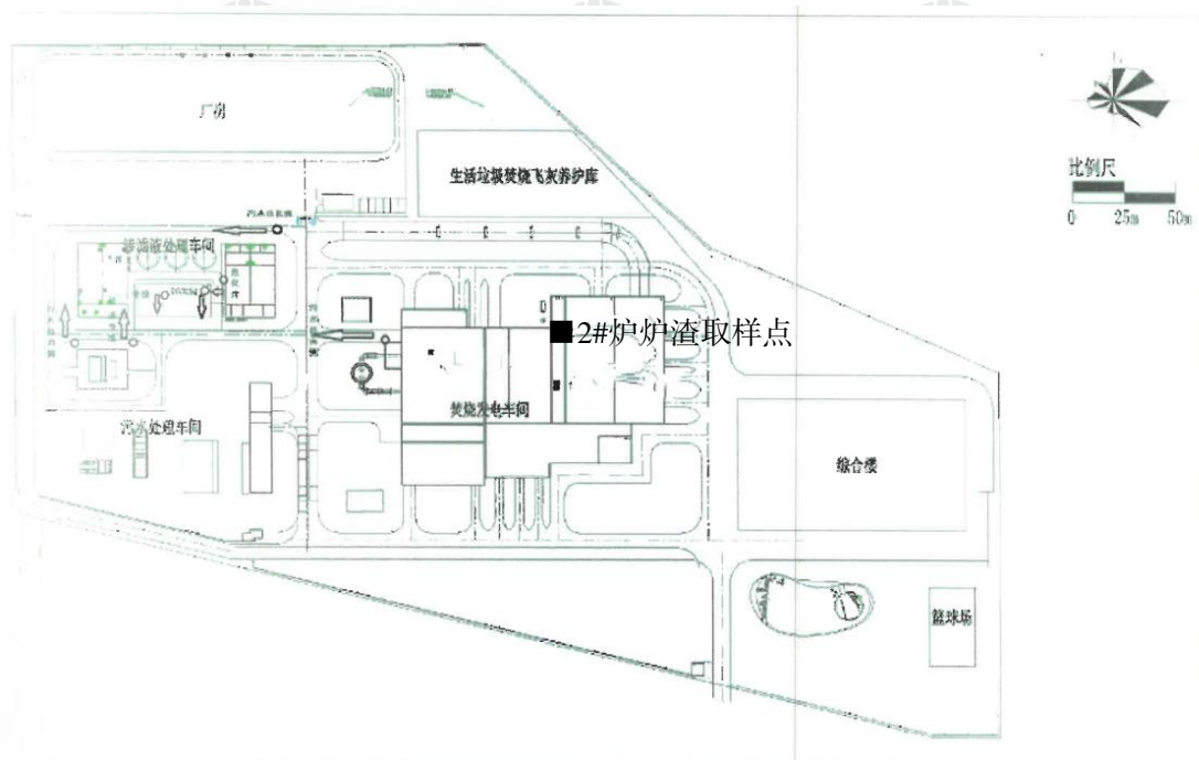
厂区平面图
